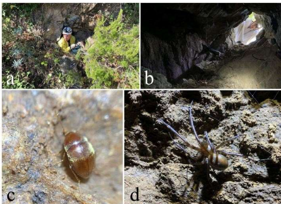
Imatges del Forat nº 1 ½ de les Pedreres. Entrada a la cavitat vista des de l'exterior (a) i des de l'interior (b); espècimen de Parvospeonomus canyellesi (c) (Coleoptera: Leiodidae); espècimen femella de Meta bournetii (d) (Arachnida: Tetragnathidae). Imatges: Jorge Mederos.
